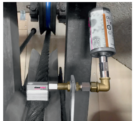
Le câble d'un téléphérique est lubrifié avec un graisseur simalube. La brosse sert à appliquer la graisse et à nettoyer le câble.
