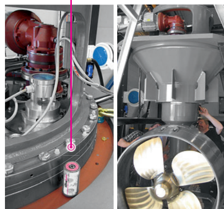
simalube 125 ml assure l'étanchéité du propulseur de poupe, pour empêcher toute entrée d'eau.
