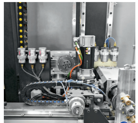
Six graisseurs fournissent le lubrifiant nécessaire aux guidages linéaires d'un centre d'usinage.
