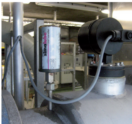
Graissage de palier à roulements : Le lubrifiant est acheminé jusqu'au palier à travers un petit tuyau.
