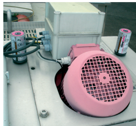
Graissage de chaînes de convoyage avec de l'huile. Les graisseurs sont disposés à l'extérieur, sur le boîtier. Un tuyau achemine l'huile jusqu'à la chaîne.
