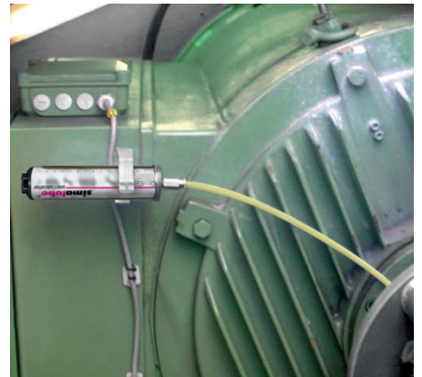
Mit dem simalube 250ml ist der Generator kontinuierlich und bis zu 12 Monaten mit Schmierstoff versorgt.
