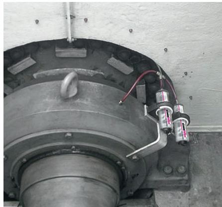
Zwei simalube 250ml schmieren das Hauptlager einer Windkraftanlage.
