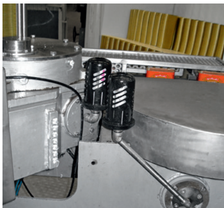
Lubricación de platos giratorios de una línea de enlatado. Los lubricadores están protegidos por una tapa de protección.
