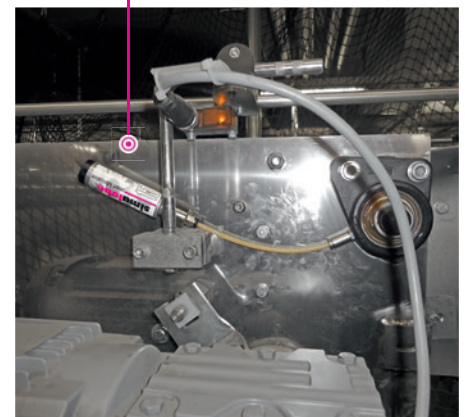
Lubricación de soportes de brida con un simalube de 15 ml, el lubricador más pequeño del mundo.
